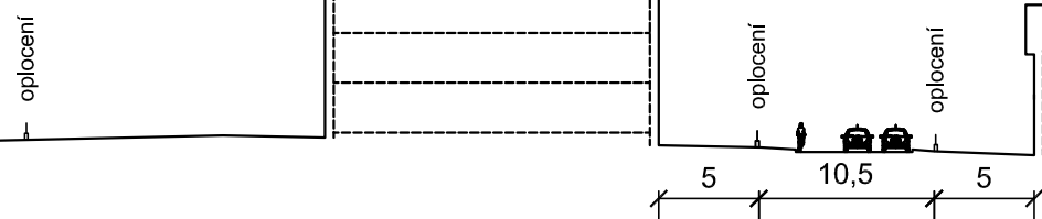
ŘEZ A-A' veřejné prostranství - ulice
